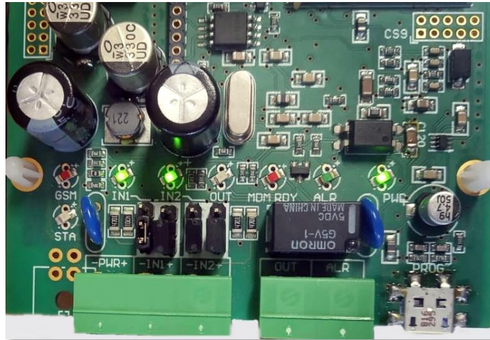
A képen a kontaktus bemenetként jumperelt bemenetek - vagyonvédelmi szenzorokhoz – láthatók (A jumperek a bemenethez közelebbi 2-tűskét zárják rövidre)
