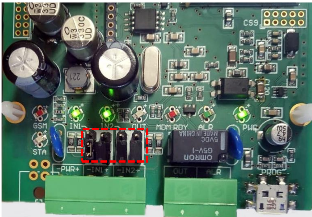
A képen a kontaktus bemenetre jumperet készülék látható (pl. vagyonvédelmi szenzorokhoz) (a jumperek ebben az esetben a bemenethez közelebbi 2 tüksén, páronként rövidre vannak zárva)
