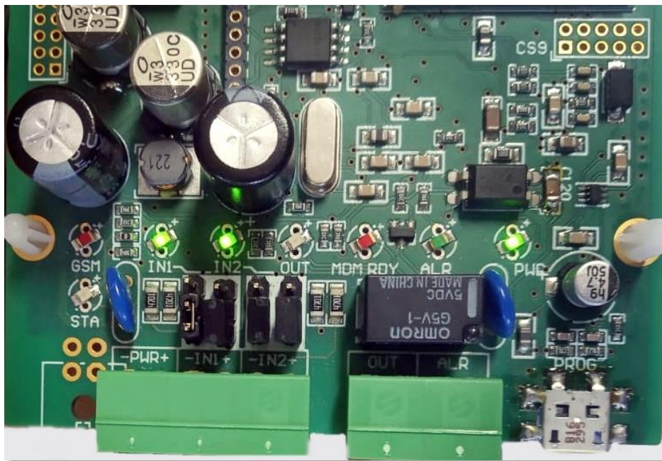
A képen a kontaktus bemenetként jumperelés látható - vagyonvédelmi szenzorokhoz – (a jumperek az alsó lábakon vannak rövidre zárva)
